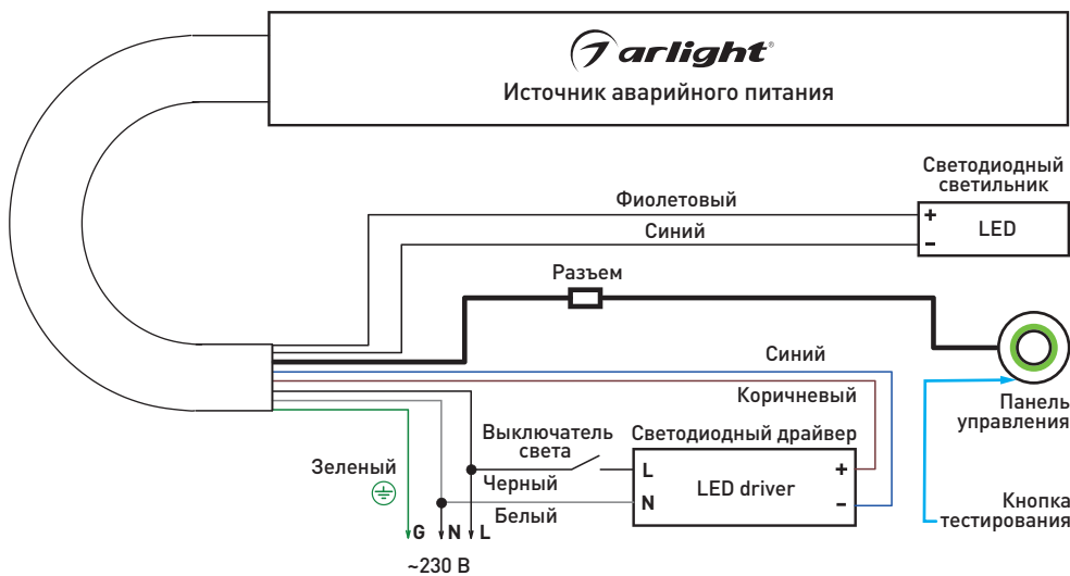
Рис. 1. Стандартная схема подключения
