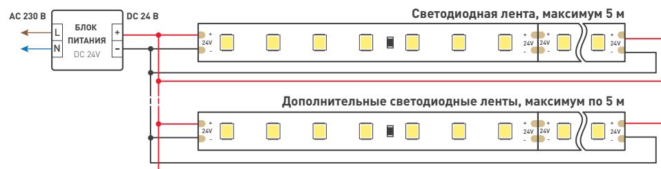
Рис. 2. Подключение нескольких светодиодных лент с двух сторон
